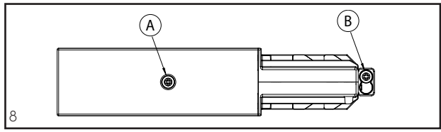
IT - Viti della testata EN - End-feed screws FR - Vis de raccord électrique DE - Schrauben Einspeisung NL - Eind fitting schroeven ES - Tornillos del cabezal NO - End-feed skruer DA - Hovedendeskrue SV - end matarskruv RU - Винты коннектора (адаптера) ZH - 端部馈电螺絲 - 端部馈电螺絲的特别之处在于它们具有特殊的形状 - AR - البراغي الخاصة بنهايات تغذية الطاقة
