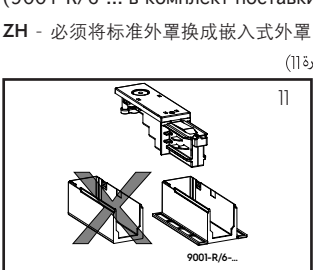
IT - Versione per controsoffitti EN - Recessed version FR - Version encastrée DE - Für die Decken Version NL - Verzonken versie - ES - Versión empotrada NO - Hengende versjon DA - Forsænket udgave SV - Infälld version RU - Версия для натяжных потолков ZH - 嵌入式版本 AR - الإصدار المُنْتَب
